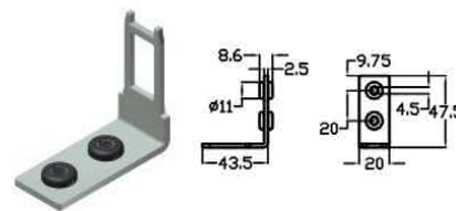
Codice ordine 27: Chiave angolare ammortizzata
