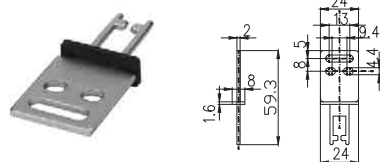
Codice ordine 46: Chiave piana
