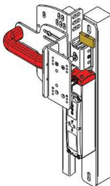
3. In presenza del lucchetto il perno di centraggio viene bloccato, non rendendo possibile l'uso del dispositivo FEP
