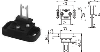
Codice ordine 49: Chiave snodata regolabile
