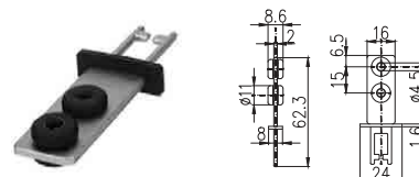
Codice ordine 8: Chiave piana ammortizzata
