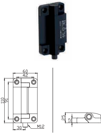
Uscita assiale inferiore con connettore M12
