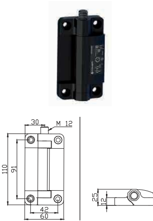
Uscita assiale superiore con connettore M12
