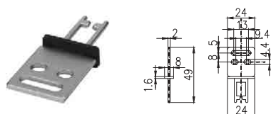
Codice ordine 6: Chiave piana
