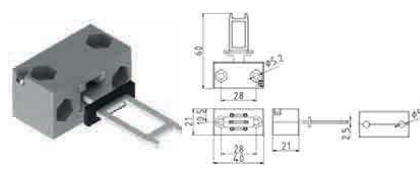
Codice ordine 29M: chiave snodata regolabile in metallo
