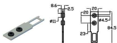
Codice ordine 28: Chiave piana ammortizzata
