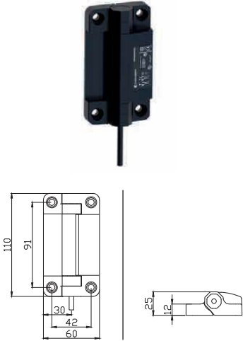
Uscita assiale inferiore
