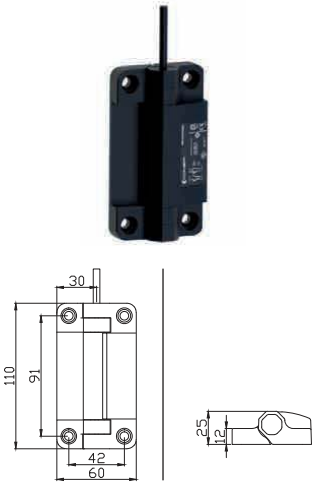
Uscita assiale superiore
