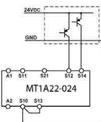
Fig. 7: Monitoraggio della protezione scorrevole a due canali cortocircuito con monitoraggio dei guasti a terra (fino alla categoria 4, PL e, SIL 3)
